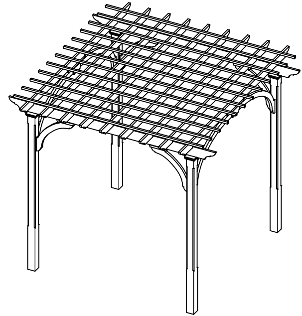
Assembled Pergola Scale: 3/16"=1'-0"
